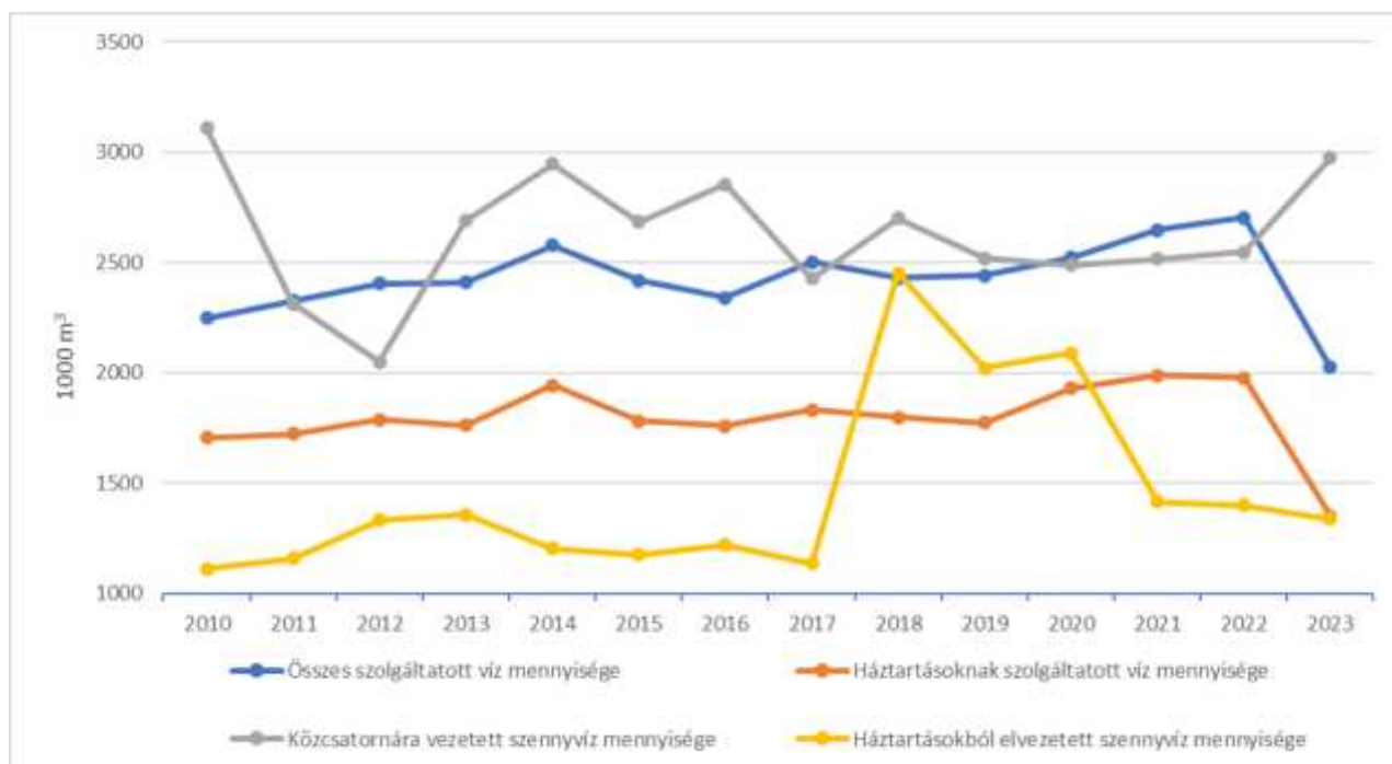
4.3.7. ábra A szolgáltatott víz és a szennyvízcsatorna-hálózatban elvezetett szennyvíz mennyiségei 2010-2023. (forrás: KSH)
